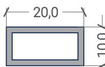
P.20x10x1,5
