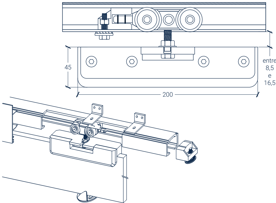
Cotas para aplicação das ferragens
